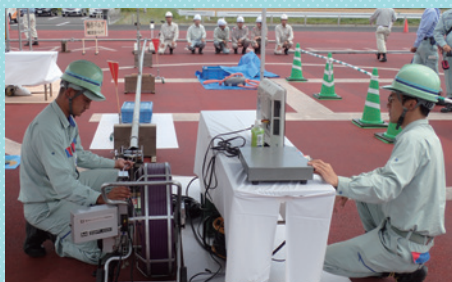
▲小型カメラをガス管に挿入し、ガス管損傷箇所を確認。
